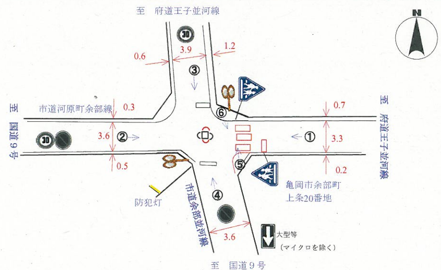
交差点図面
