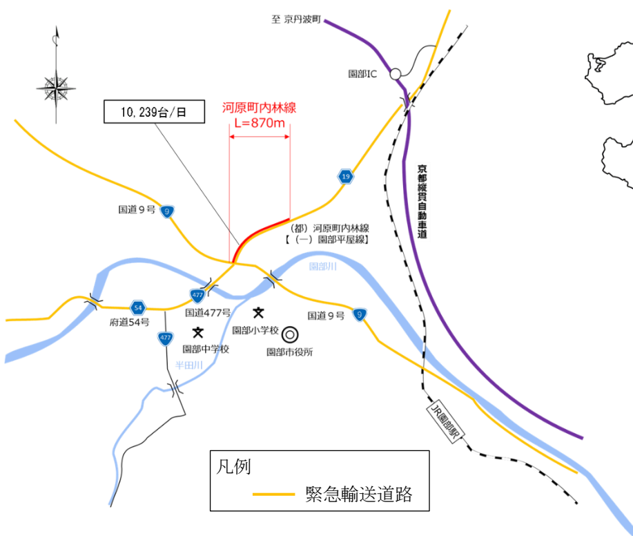
位置図 (詳細)
