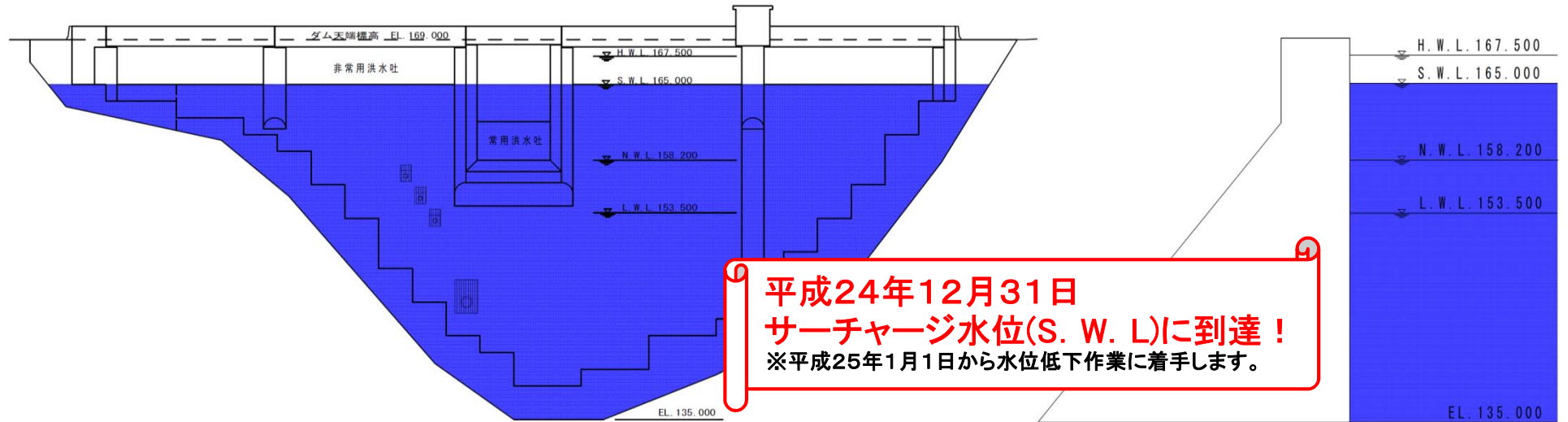
(畑川ダム上流面図)
