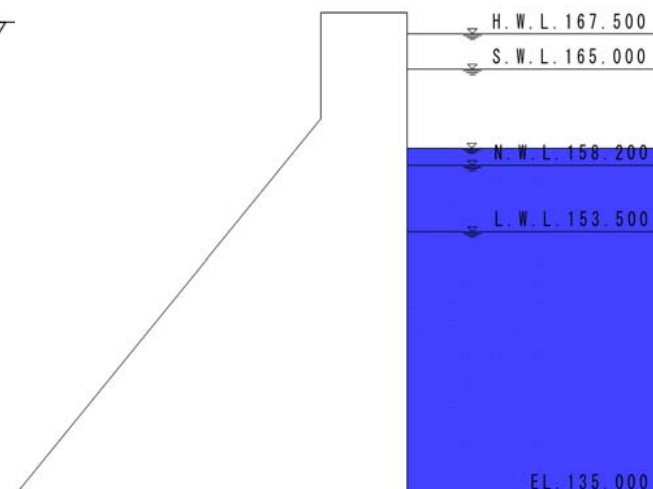
(畑川ダム断面図)
