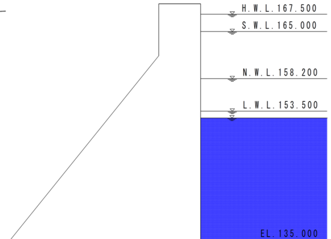
(畑川ダム断面図)
