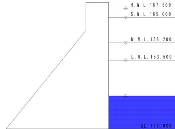
(畑川ダム断面図)
