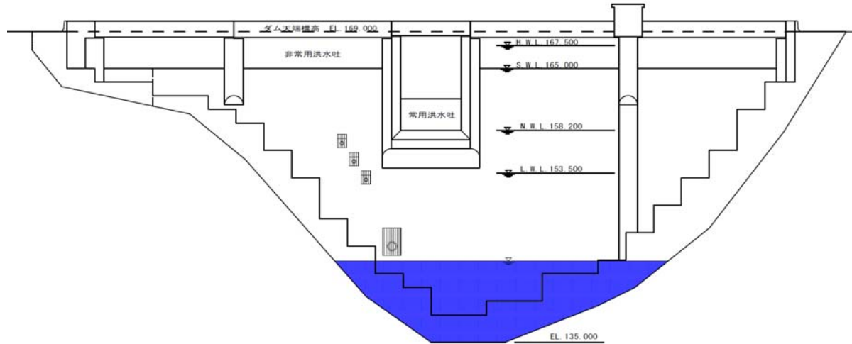
(畑川ダム上流面図)
