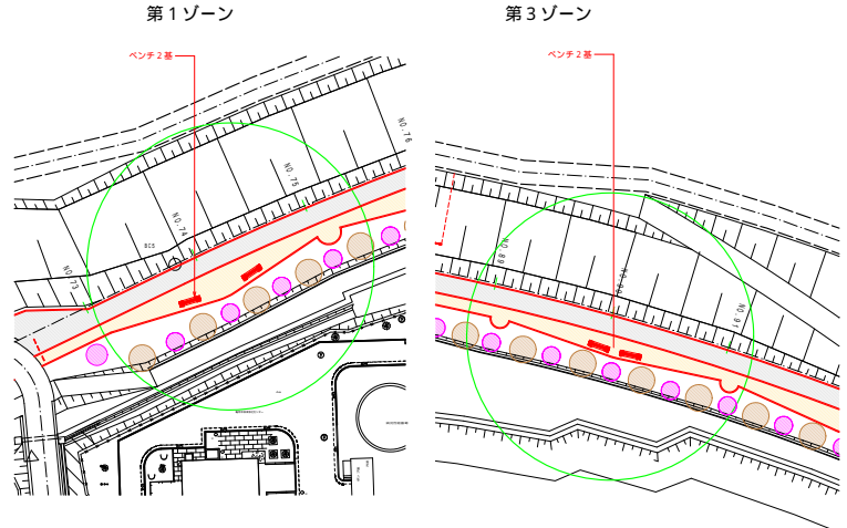
施設部平面図 S=1:500 (拡大図)
