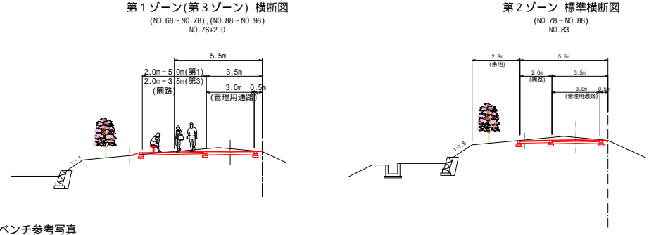
代表横断面 S=1:100
