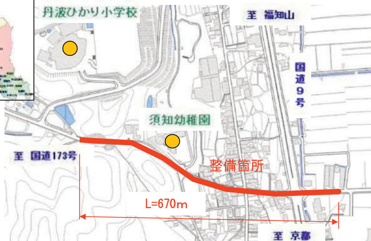
平面図
