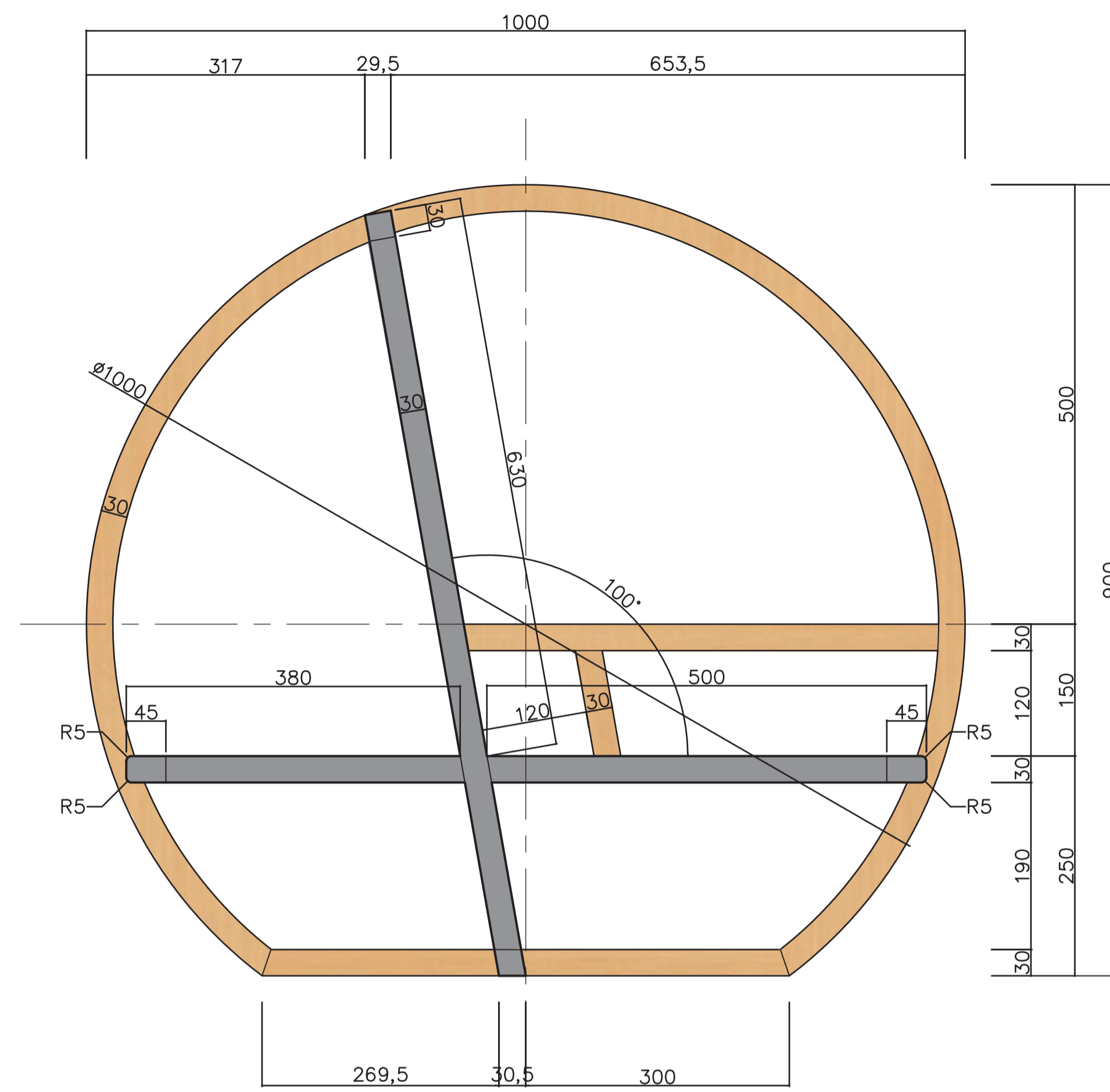
A-A'断面図 S=1:5
