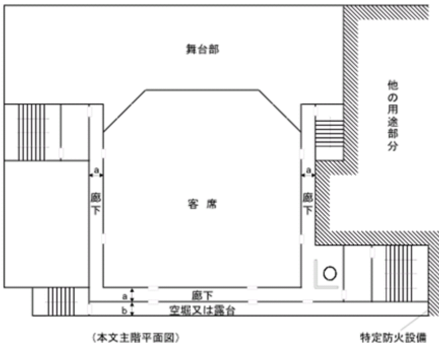
(図 11 一主階が避難階以外にある興行場等)
