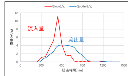
堰堤の流入流出
