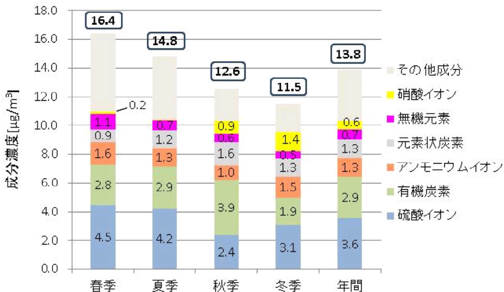
図3-19 PM 2.5 成分分析結果
