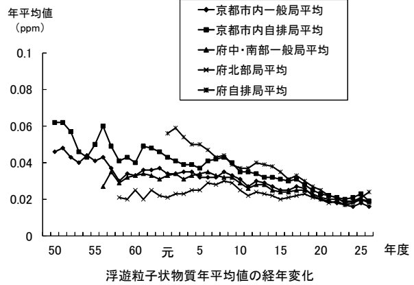
図3-20 環境基準が定められている物質の年平均値の経年変化等
