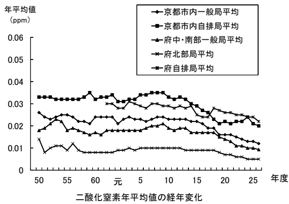
図3-20 環境基準が定められている物質の年平均値の経年変化等
