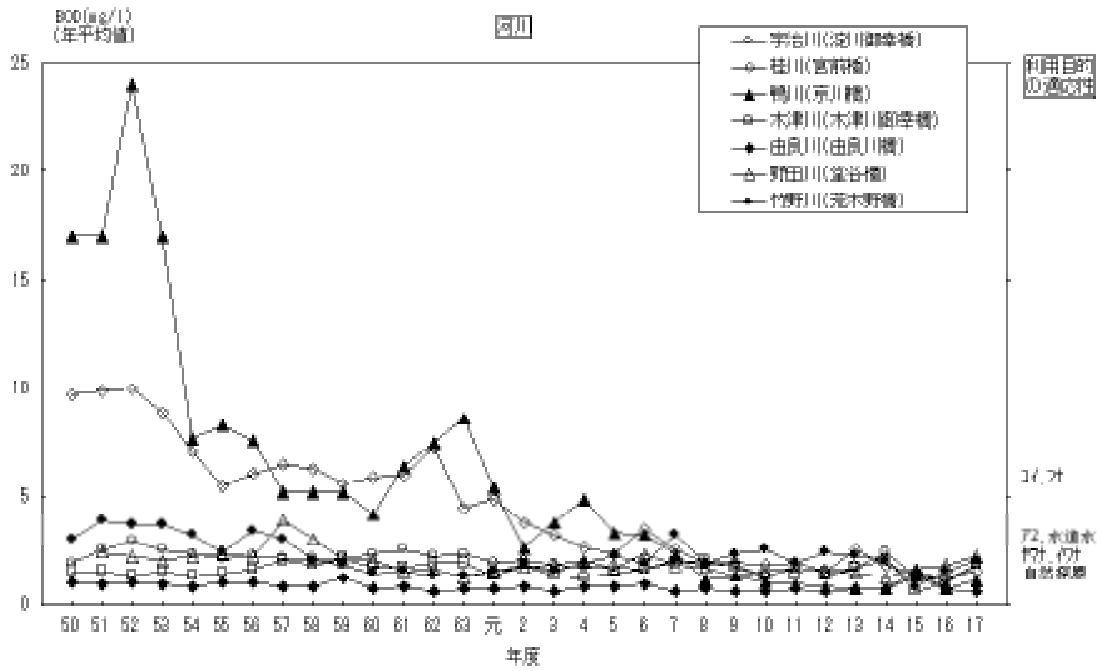
図3-15 主要環境基準点（河川）のBODの年次推移
