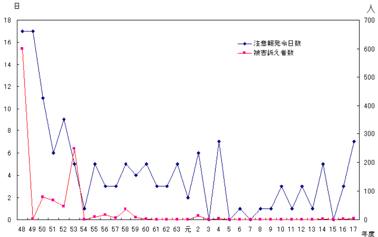
図3-12 光化学スモッグ注意報発令状況
