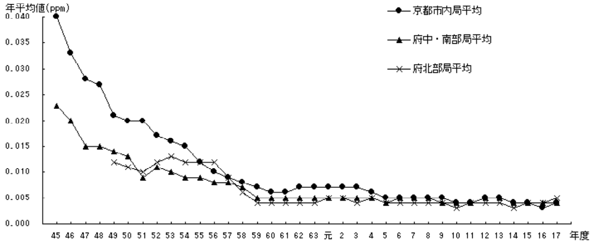
図3-14 一酸化炭素の年平均値の経年変化
