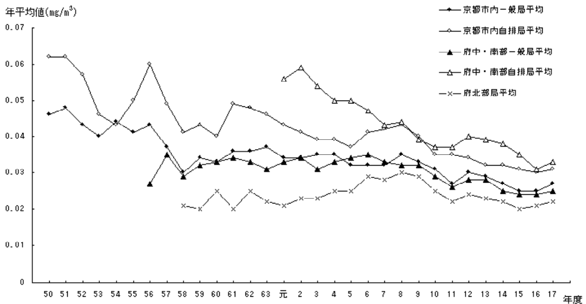
図3-11 浮遊粒子状物質の年平均値の経年変化
