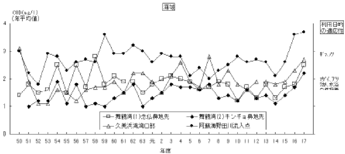
図3-16 主要環境基準点（海域）のCODの年次推移
