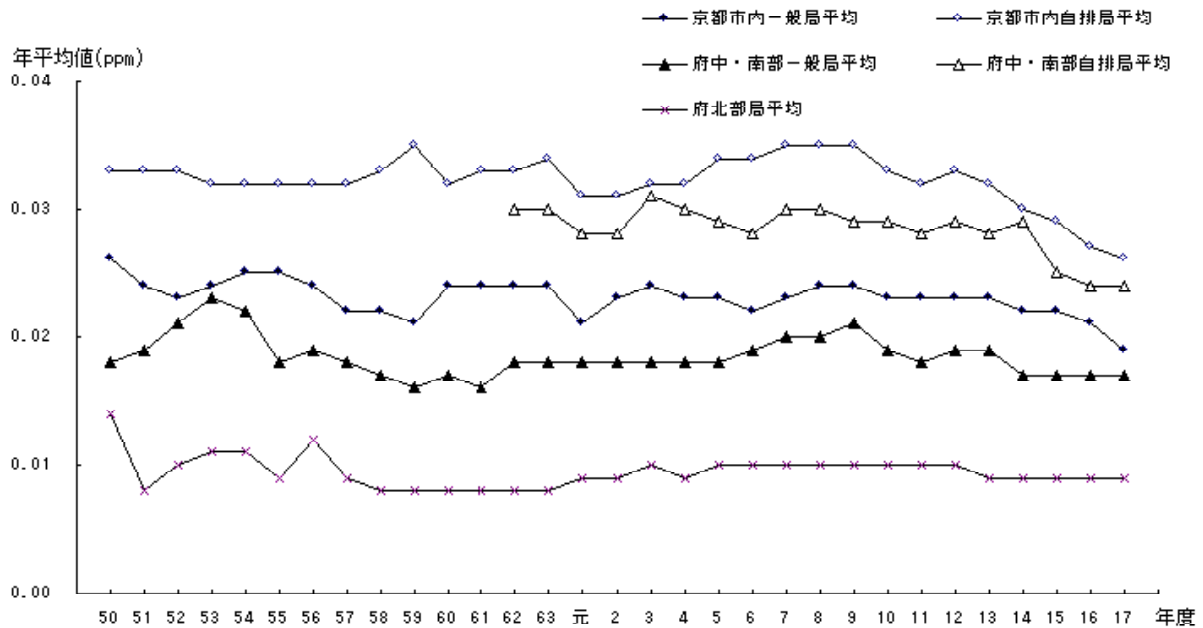
図3-10 二酸化窒素の年平均値の経年変化
