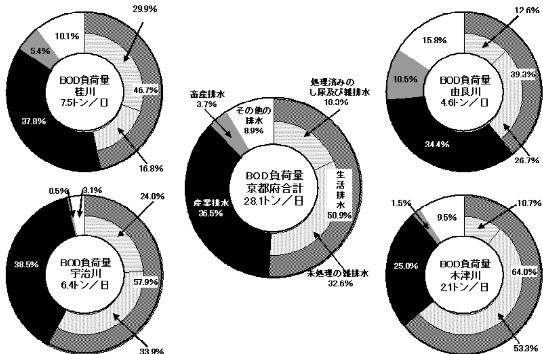
図3-17 BOD負荷量の発生源別割合（17年度）
