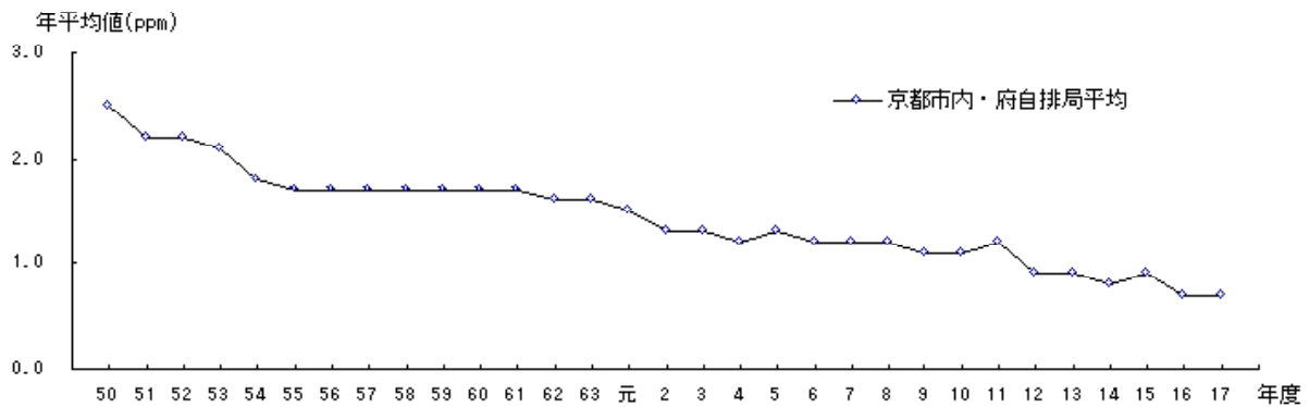
図3-14 一酸化炭素の年平均値の経年変化
