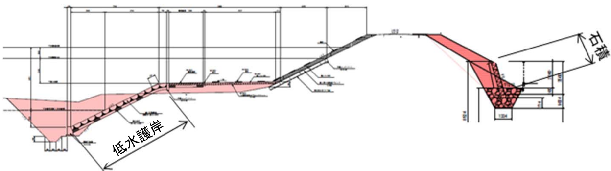
標準断面図
