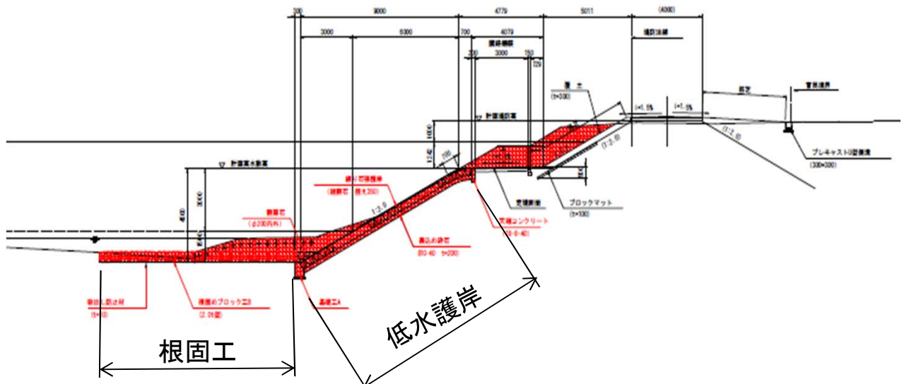
標準断面図
