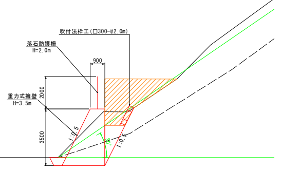
標準断面図
