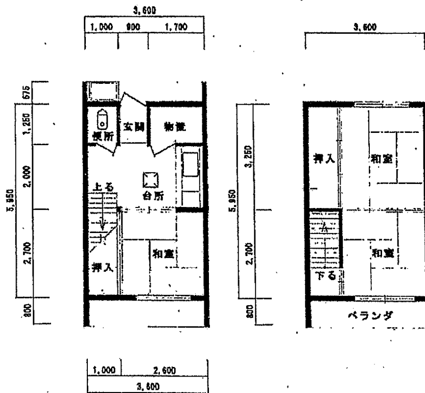
1 階平面図
