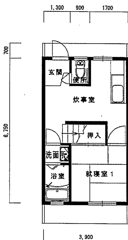
1階平面図
