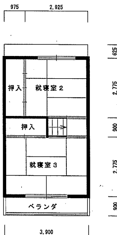
2階平面図
