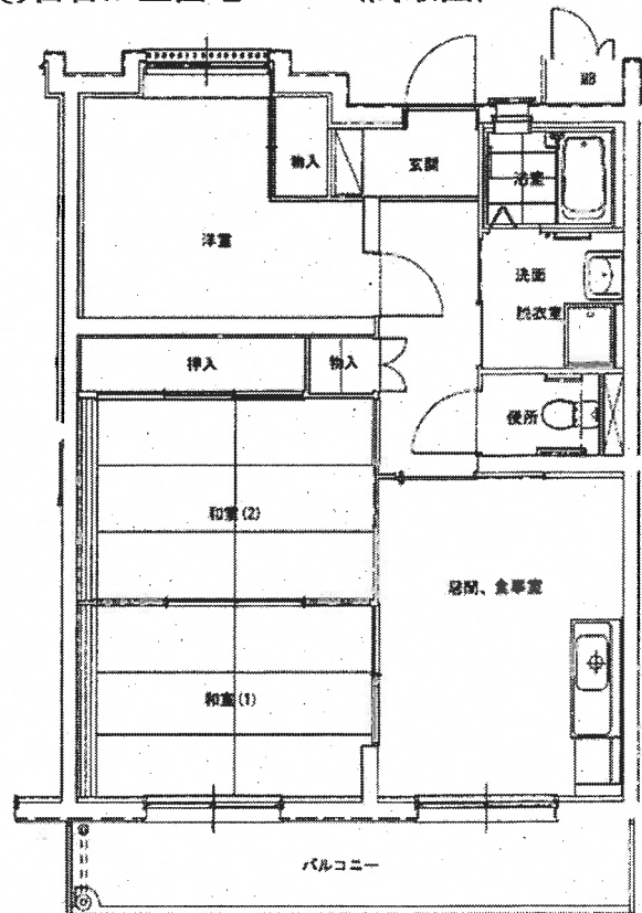
③⑫百合が丘団地 3DK (間取図)
