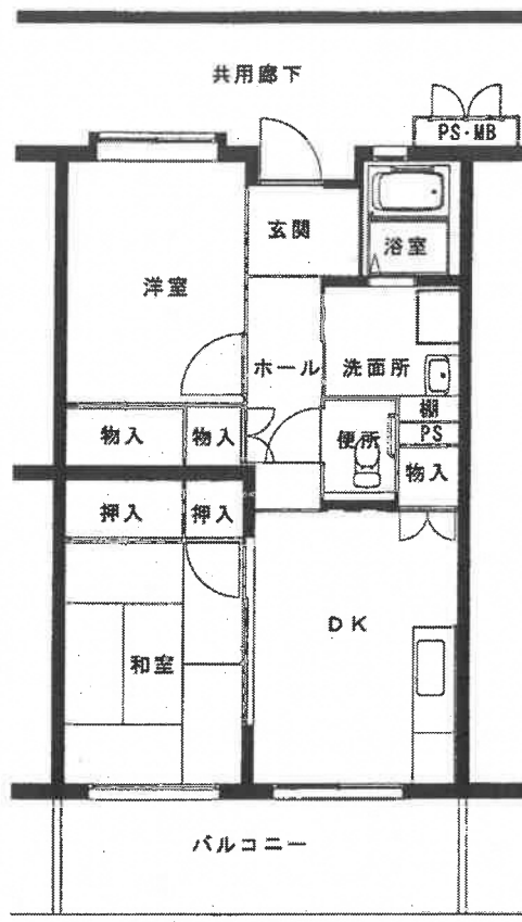
③明石団地 2DK (間取図)
