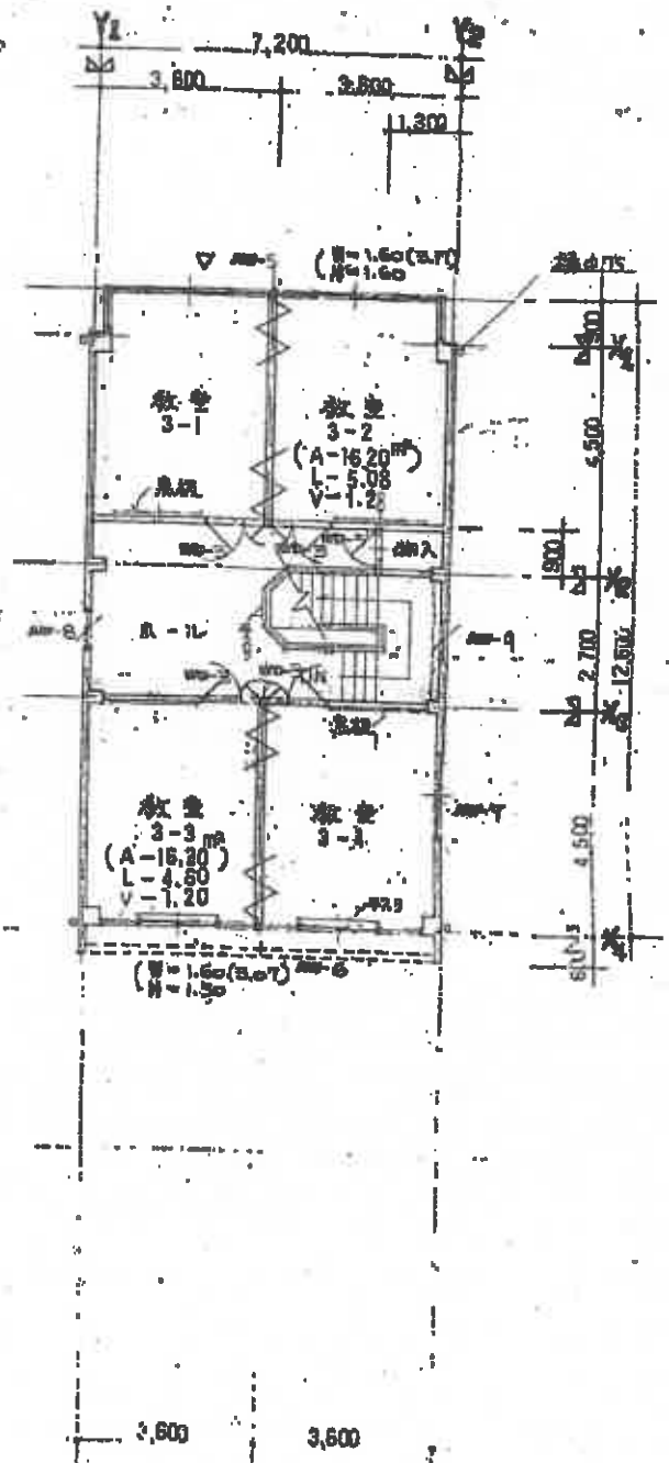
3F 平面図 1/100 A 3 - 80.72 m 2
