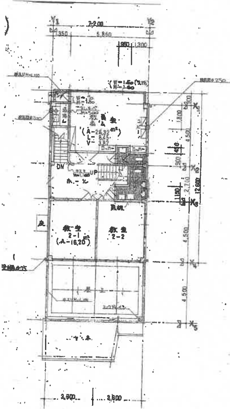
2F 平面図 1/100 A 2 - 89.51 m 2
