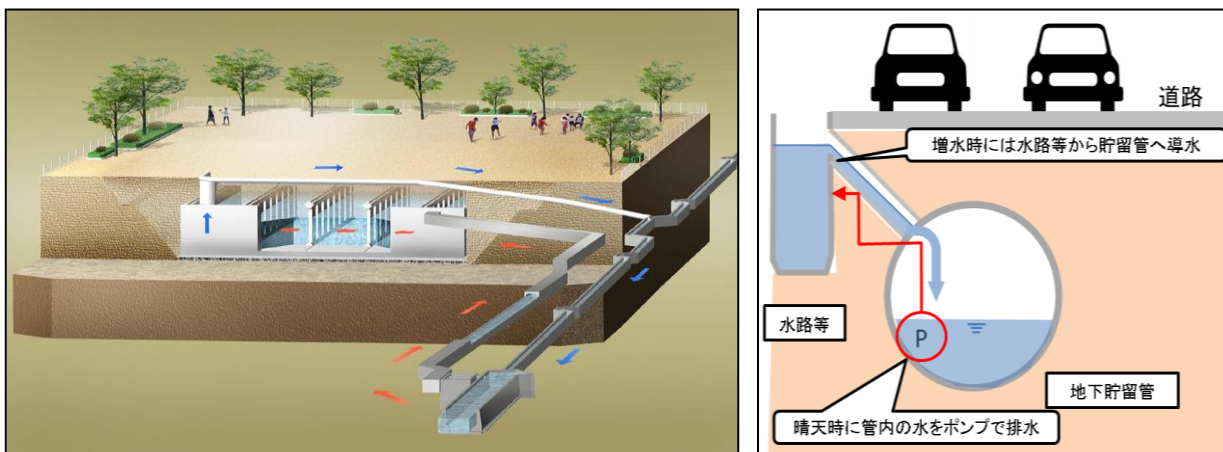
図－1 雨水地下貯留施設、雨水地下貯留管の例
