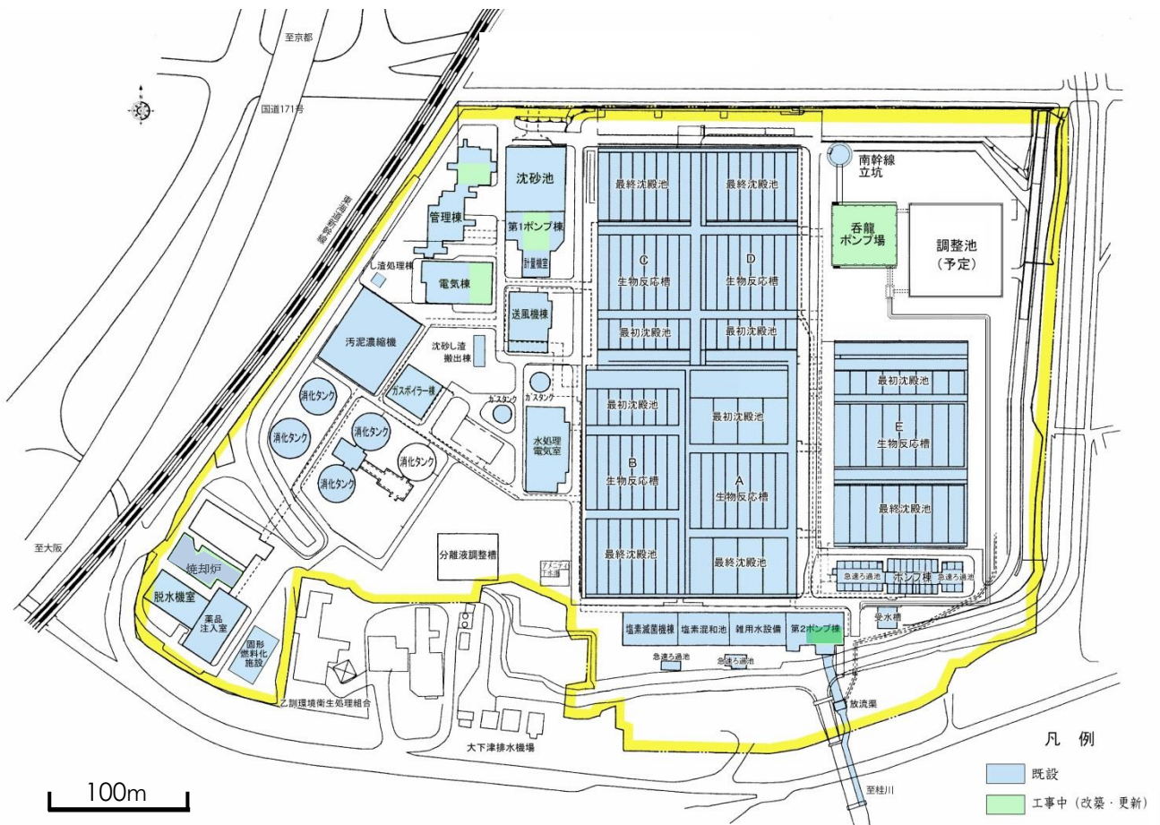
洛西浄化センター平面図
