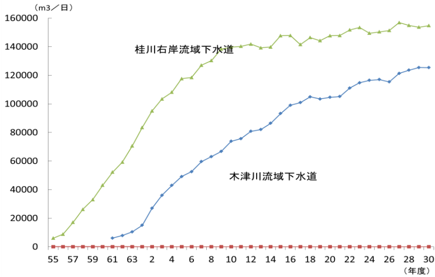
日平均流入水量の推移
