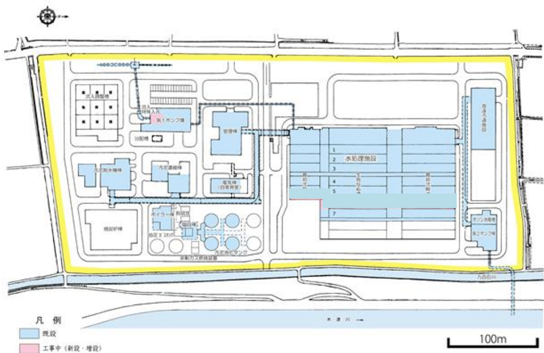
木津川上流浄化センター平面図
