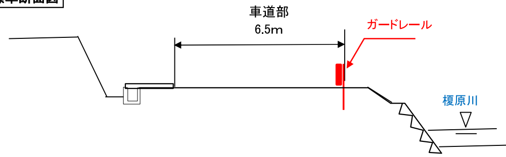
標準断面図
