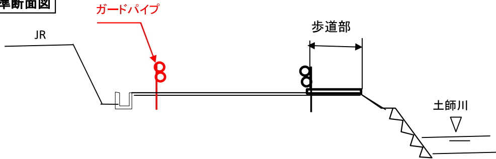
標準断面図
