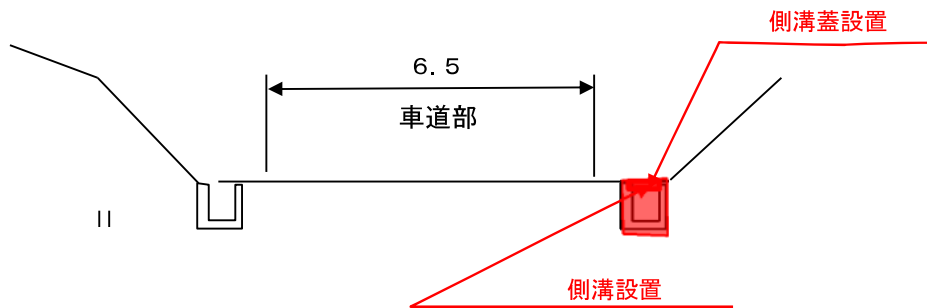
標準断面図
