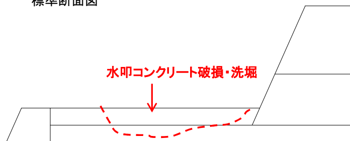
標準断面図
