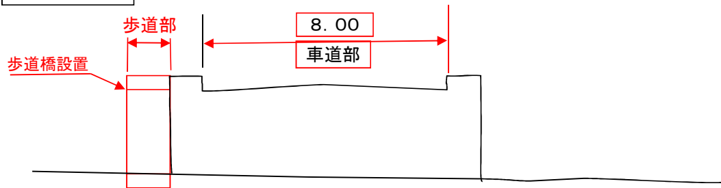
標準断面図
