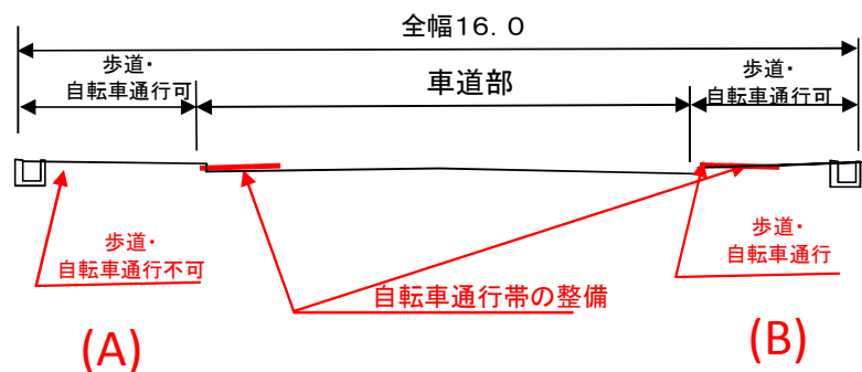
標準断面図
