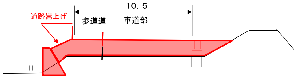
標準断面図
