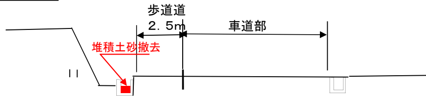
標準断面図
