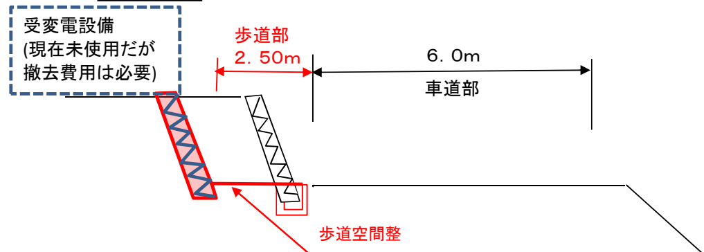
標準断面図
