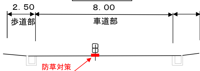
標準断面図
