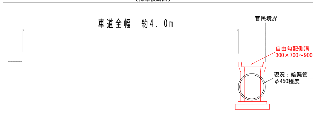
〔標準横断面〕
