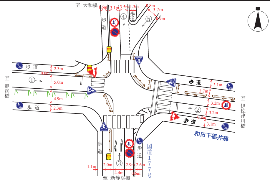
交差点図面
