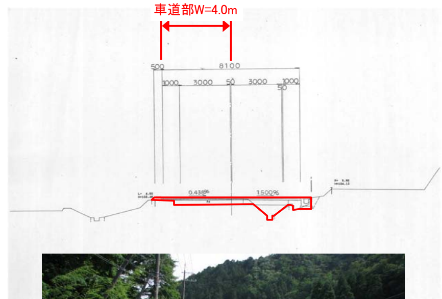
〔標準横断面図〕
