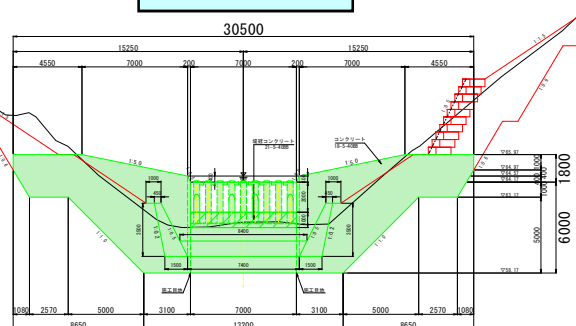
堰堤断面図
