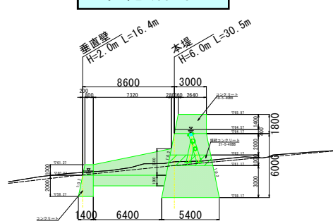
堰堤断面図
