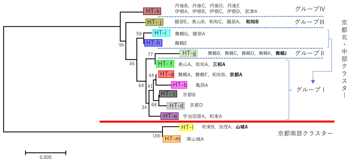
図 1-2 ミトコンドリア DNA の塩基配列に基づく分子系統樹
