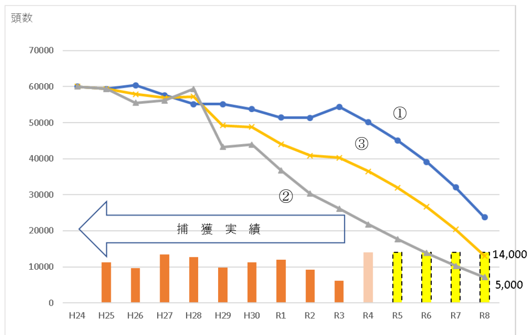
図3 推定生息数のシミュレーション 平成24年度時点の推定生息数を60,000頭として算出した暫定値
