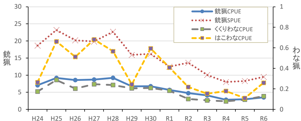
図1 捕獲効率（CPUE）及び目撃効率（SPUE）の推移
