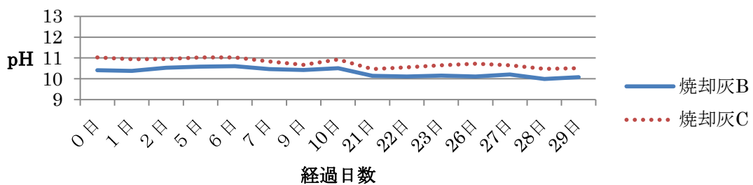
焼却灰の屋外放置における pH の推移
